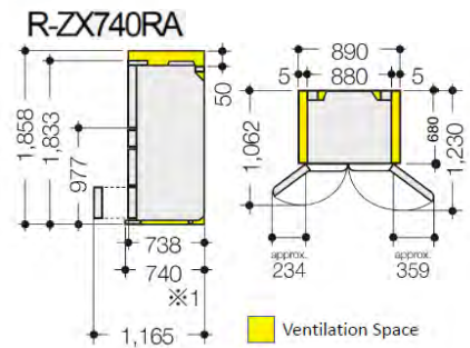
Dimensions 1833(h) x 880(w) x 738(d) mm
